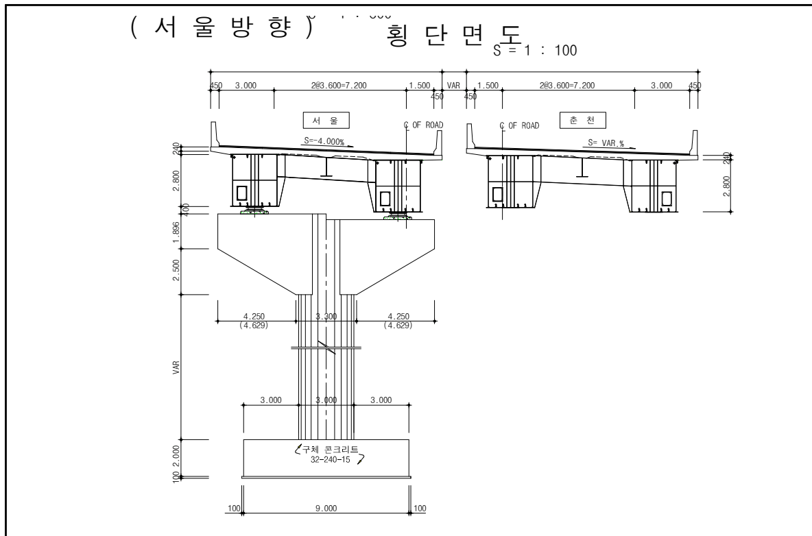
【그림 1.3】 군자4교(서울) 횡단면도
