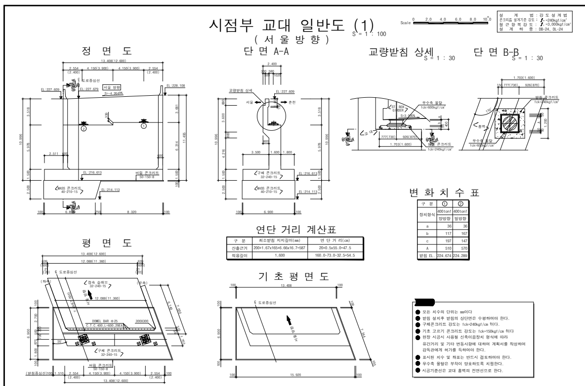
【그림 1.4】 군자4교(서울) 시점교대 일반도
