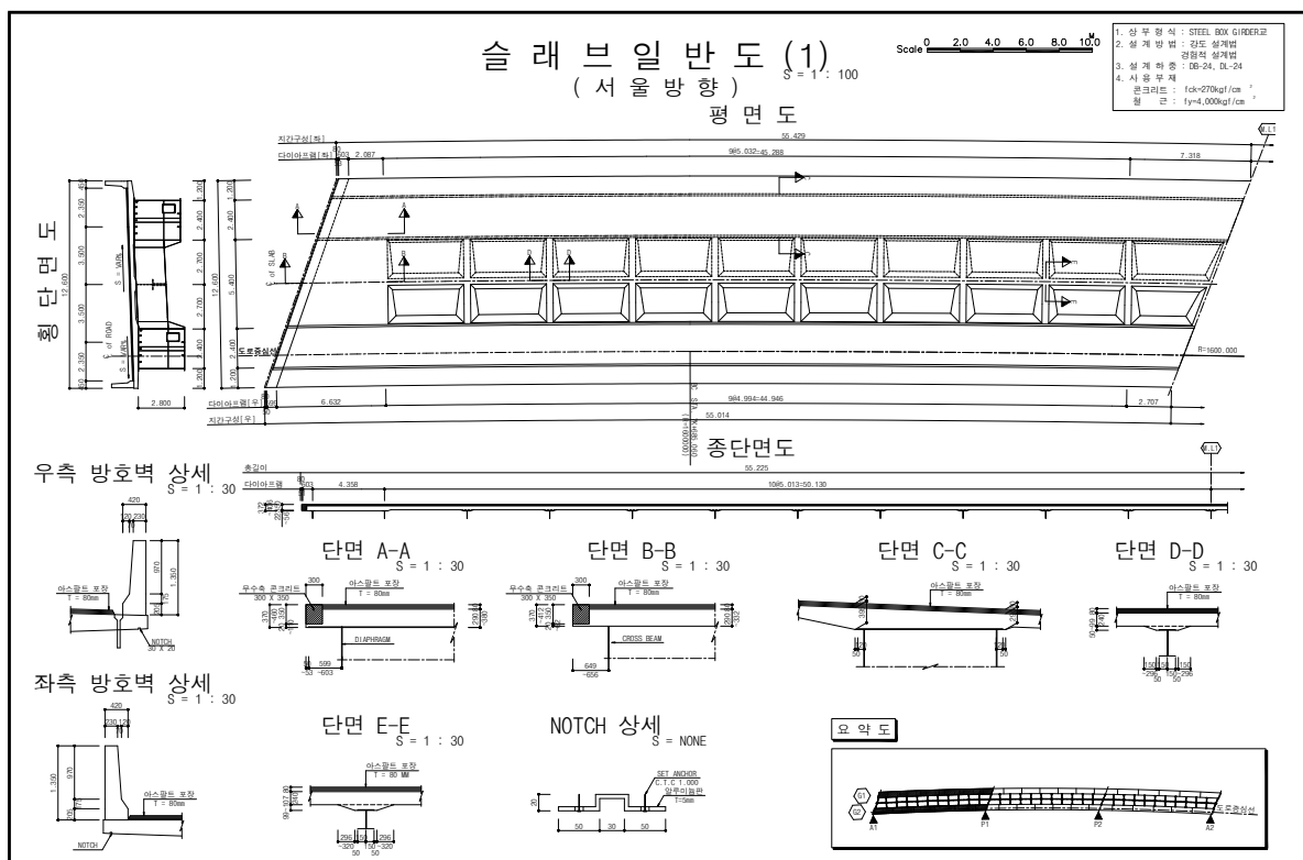
【그림 1.6】 군자4교(서울) 슬래브 일반도
