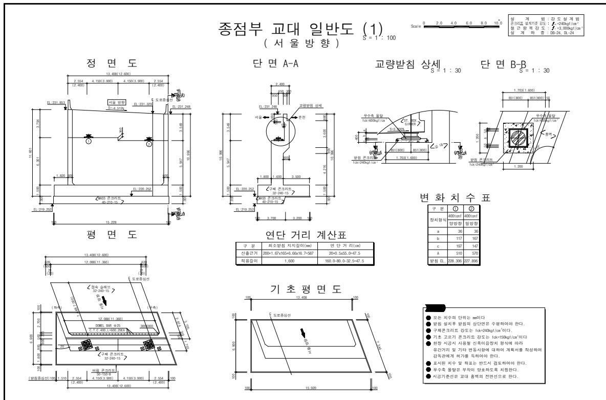
【그림 1.5】 군자4교(서울) 종점교대 일반도
